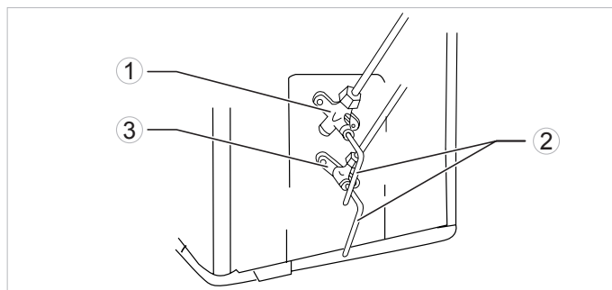
Afb. 12.6 Openen van de tweeweg- en driewegkleppen.
