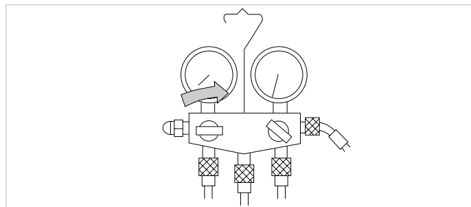
Afb. 12.4 Aanduiding van de lagedrukmanometer met gesloten klep "Low": opsporen van lekken.
