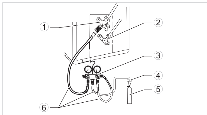
Afb. 12.1 Opsporen van lekken in de installatie.
