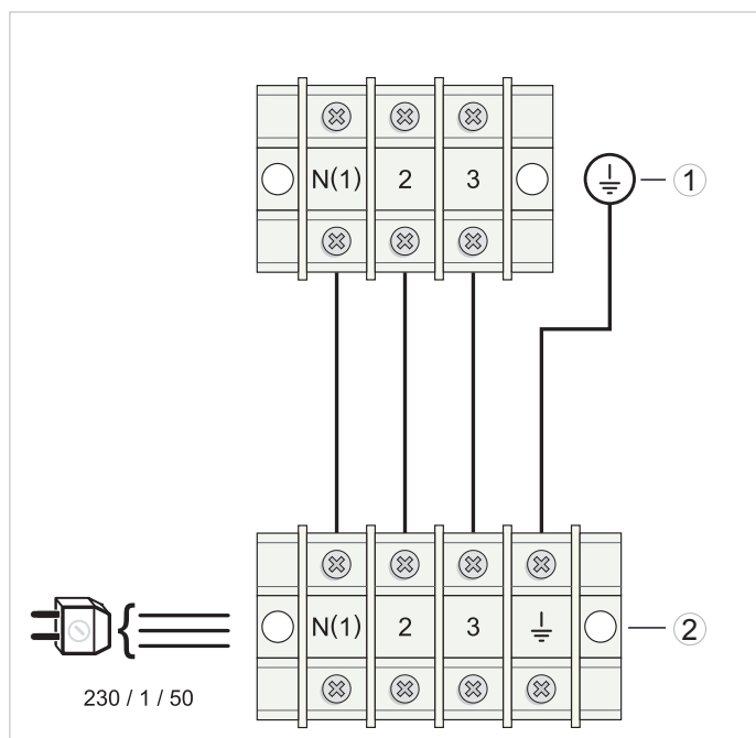
Afb. 11.4 Elektrisch verbindingsschema tussen de externe en binnenuit SDH 18-025 NW en SDH 18-035 NW.
