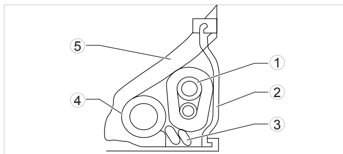
Afb. 9.10 Leggen van de leidingen.
