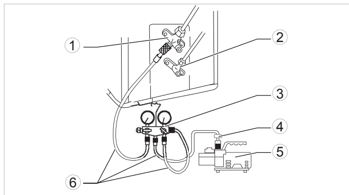
Afb. 12.2 Ledigen van de installatie
