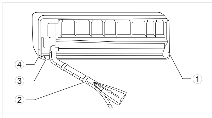
Afb. 9.8 Vensters voor het installeren van de leidingen.
