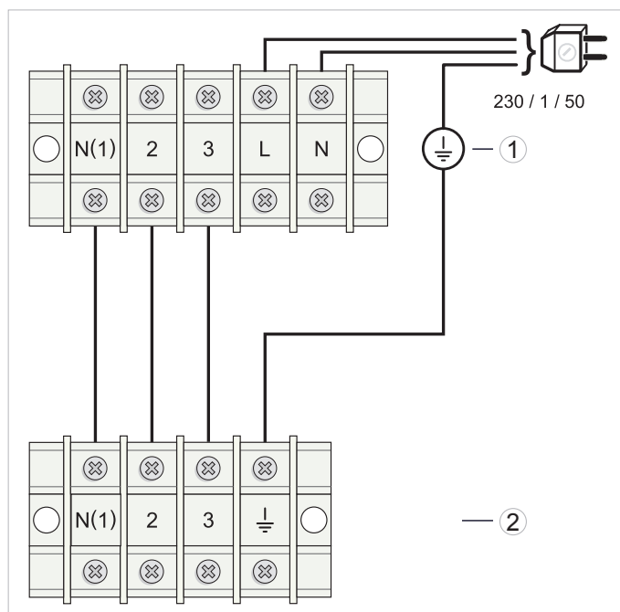
Afb. 11.5 Elektrisch verbindingsschema tussen de externe en Binnenuit SDH 18-050 NW en SDH 18-035 NW.
