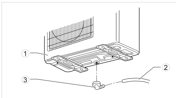
Afb. 10.1 Montage van de elleboog voor condensatiewaterafvoer.
