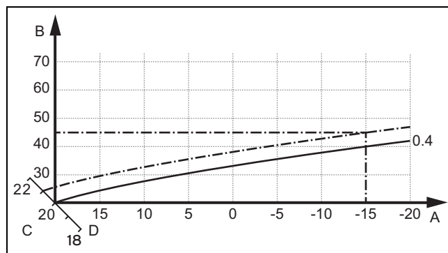
A Température extérieure en °C C Température ambiante de consigne en °C B Température de départ de consigne en °C D Axe a
